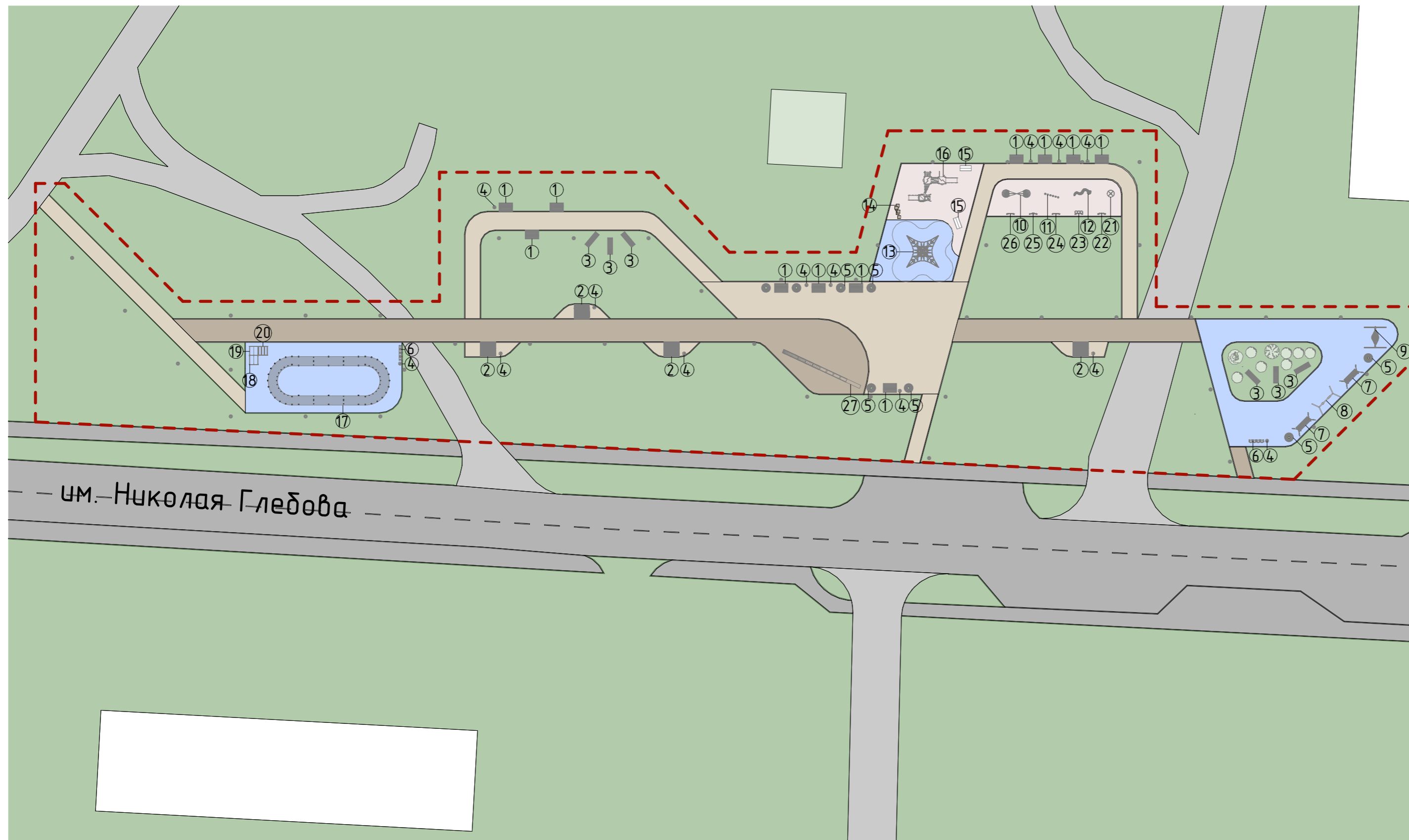
Схема генплана
